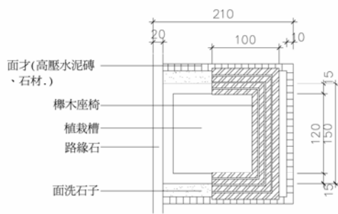
植栽槽平面圖
