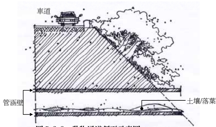
圖 5-2-3、動物通道剖面示意圖
