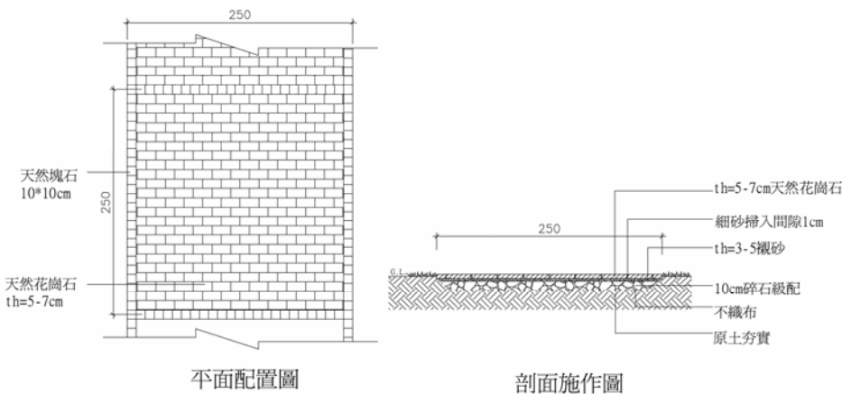
石材人行道剖面施作圖(乾式)
